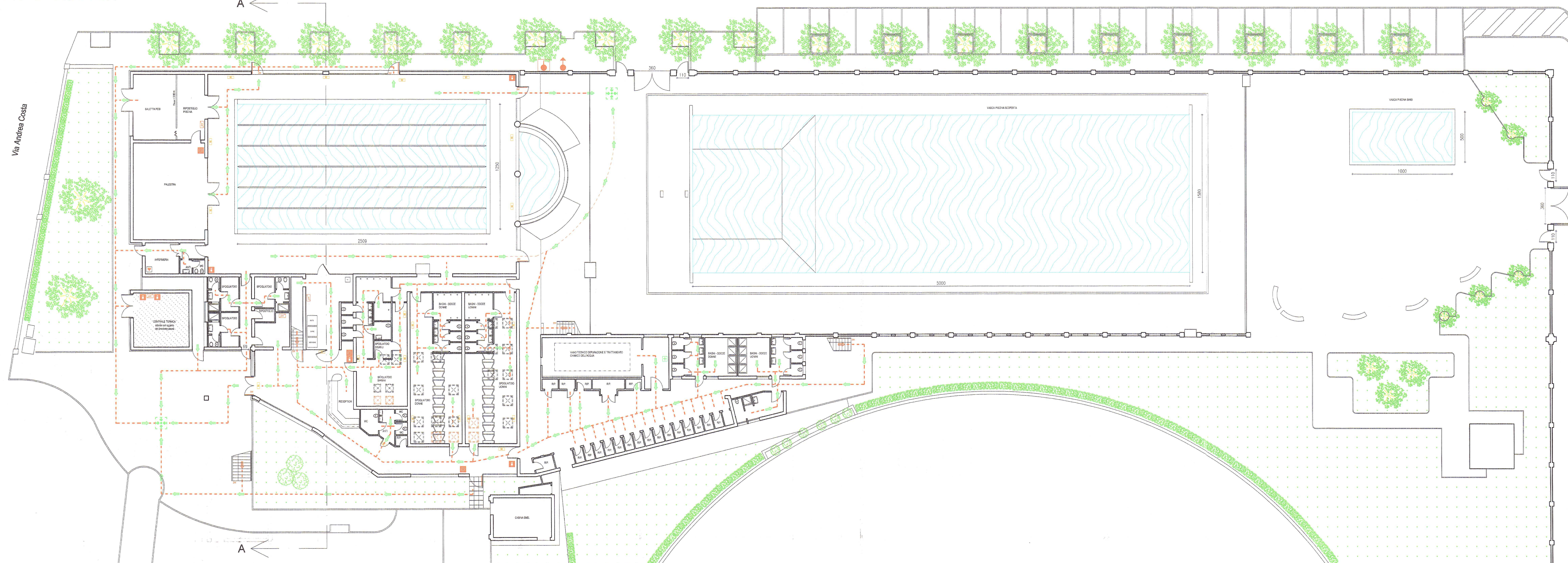
Piscine Comunali di Molinella Piano Terra - Scala 1:200
